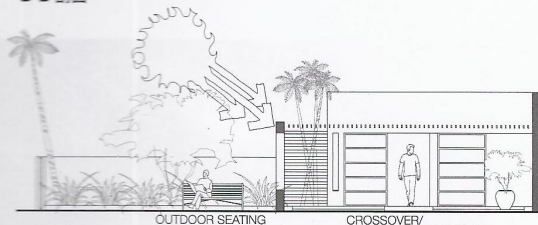
C-C 剖面
