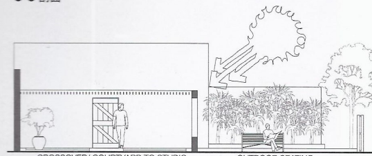
D-D 剖面
